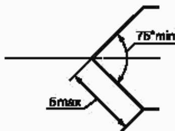
Рисунок 1 — Угол схождения боковых граней острия клинка
